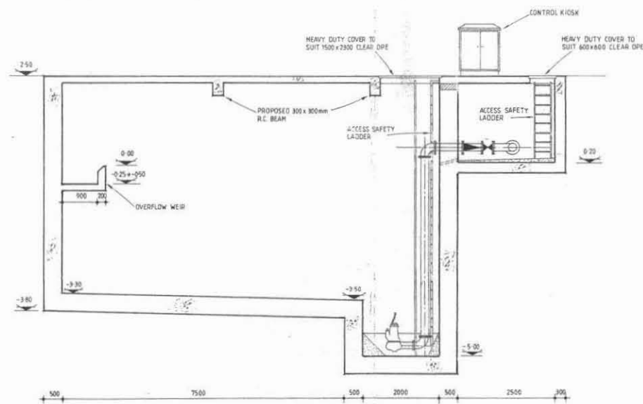
SECTION A-A 1/50
