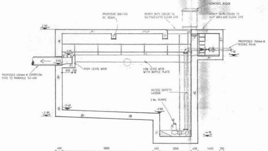
SECTION A-A 1/50
