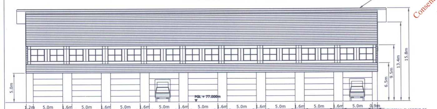
ELEVATION A
