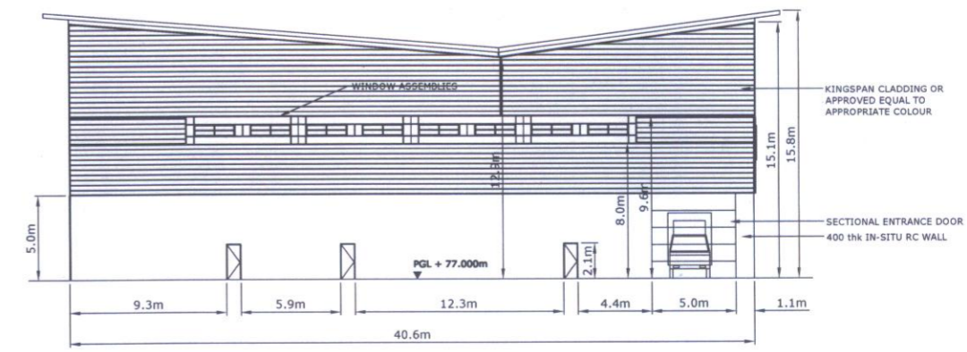
ELEVATION B
