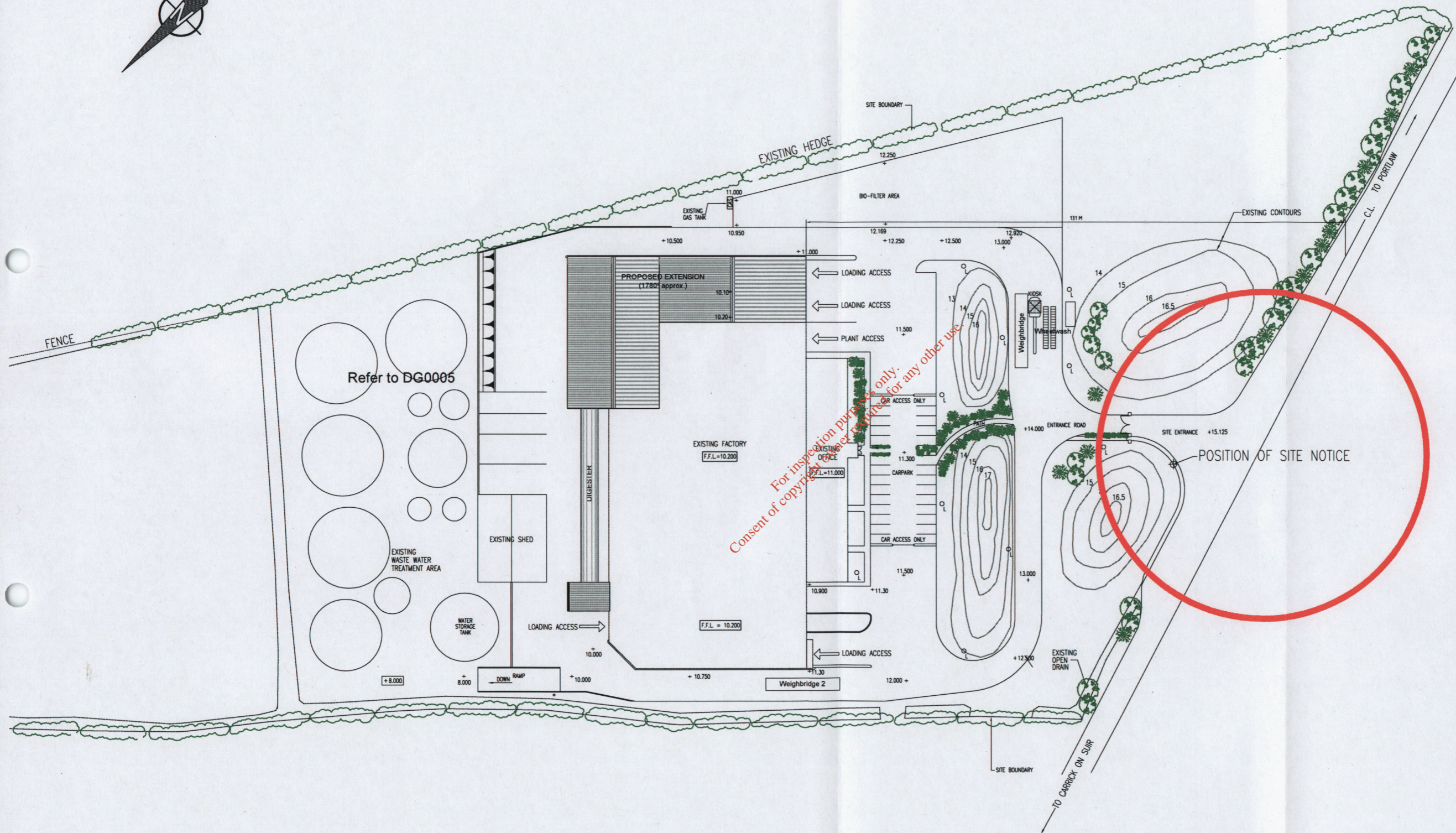
SITE LAYOUT (1:500)
