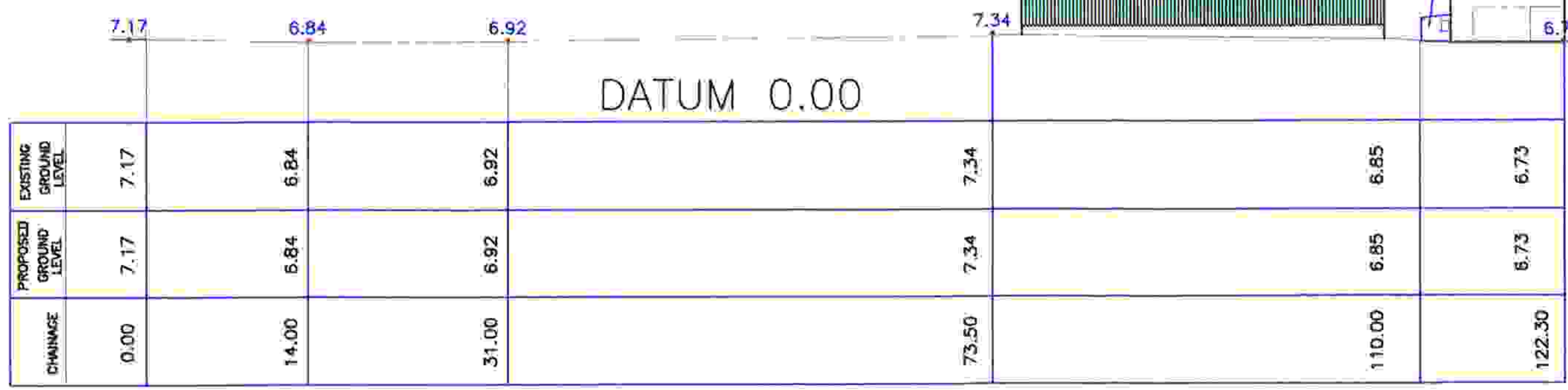
SITE SECTION B - B
